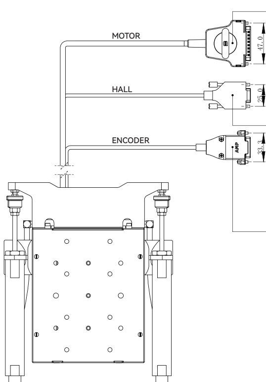
XAZS130P-T03/T06-U04R4A1-D2-MS PIN OUT
