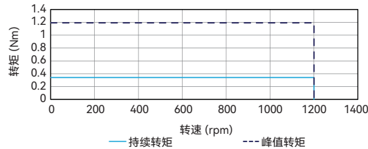
转矩-转速曲线 ACD62-P-30 三角形接法 直流母线电压 48V
