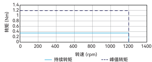
转矩-转速曲线 ACD62-P-30 星形接法 直流母线电压 48V
