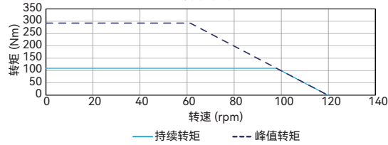
转矩-转速曲线 ADR320-P-80 串联接法 直流母线电压 600V
