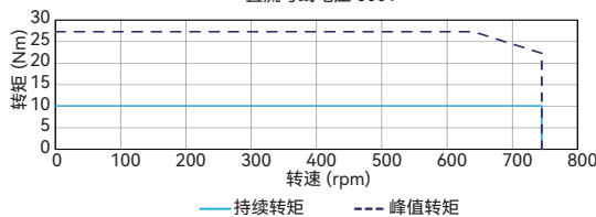
转矩-转速曲线 ADR135-P-54 并联接法 直流母线电压 330V
