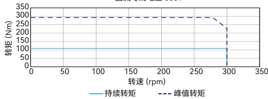
转矩-转速曲线 ADR320-P-80 并联接法 直流母线电压 600V
