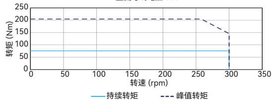
转矩-转速曲线 ADR220-P-100 并联接法 直流母线电压 600V
