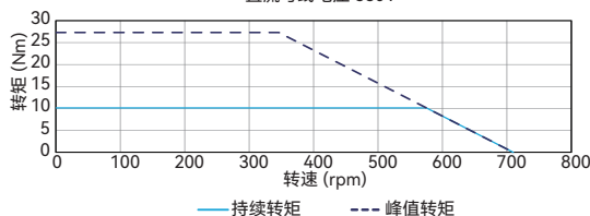
转矩-转速曲线 ADR135-P-54 串联接法 直流母线电压 600V
