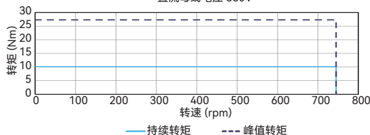
转矩-转速曲线 ADR135-P-54 并联接法 直流母线电压 600V
