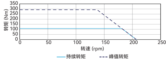
转矩-转速曲线 ADR320-P-80 并联接法 直流母线电压 330V
