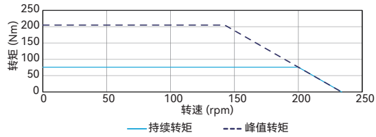
转矩-转速曲线 ADR220-P-100 并联接法 直流母线电压 330V
