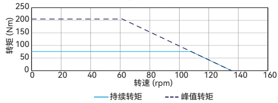
转矩-转速曲线 ADR220-P-100 串联接法 直流母线电压 600V
