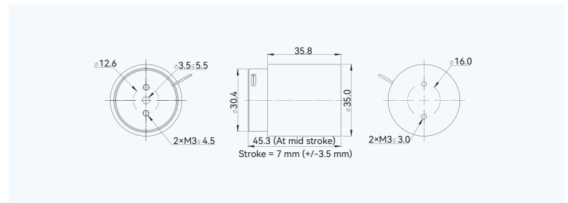
■ 尺寸图
