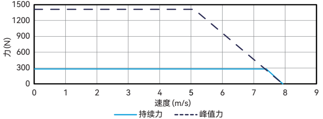
力速曲线 ALM048-T-B2-H 直流母线电压 330V
