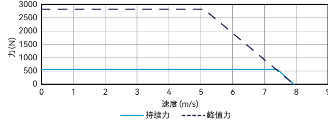
力速曲线 ALM048-T-B4-H 直流母线电压 330V
