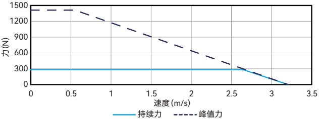
力速曲线 ALM048-T-B2-M 直流母线电压 330V
