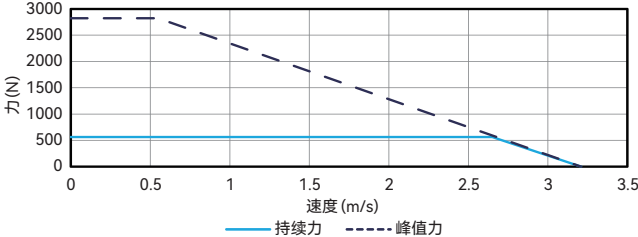
力速曲线 ALM048-T-B4-M 直流母线电压 330V
